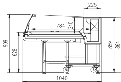
HORIZONTAL WITH LOW SELF-SERVICE GLASS HORIZONTAL MIT SELBSTBEDIENUNGSSCHEIBEN ВИТРИНА В РАЗЛОЖЕННОМ ВИДЕ - НИЗКОЕ СТЕКЛО - САМООБСЛУЖИВАНИЕ
