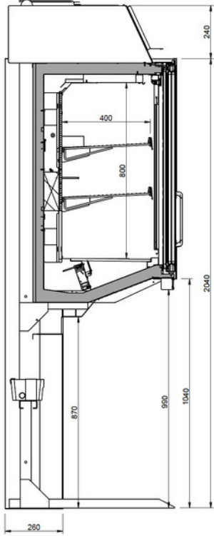
LINEAR CABINET
